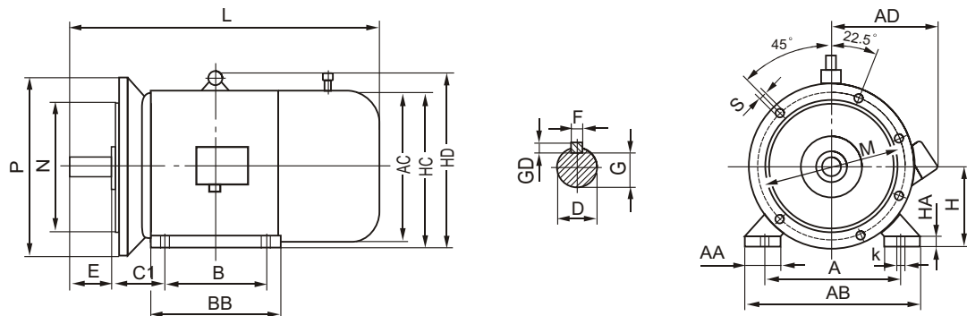
图3 YEJ系列（B35）（见表5） Figure 3 YEJ Series（B35）（See table 5）
